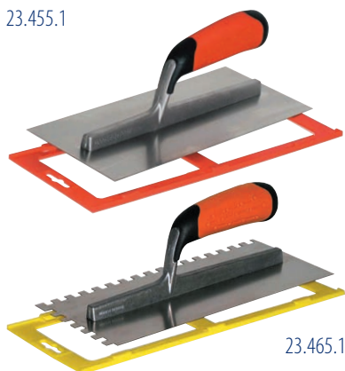
Стальные гладилки. Лезвия: прямые заточенные или зуб- чатые. 28x12 см и 35x10 см
