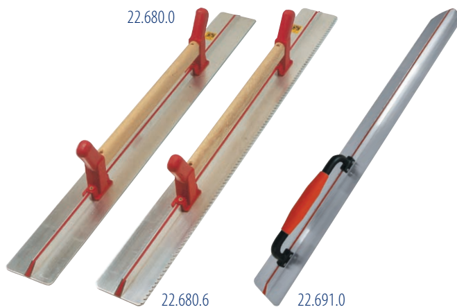
Алюминиевые двуручные правила для стен. Длина: от 0,8 м до 1,2 м
